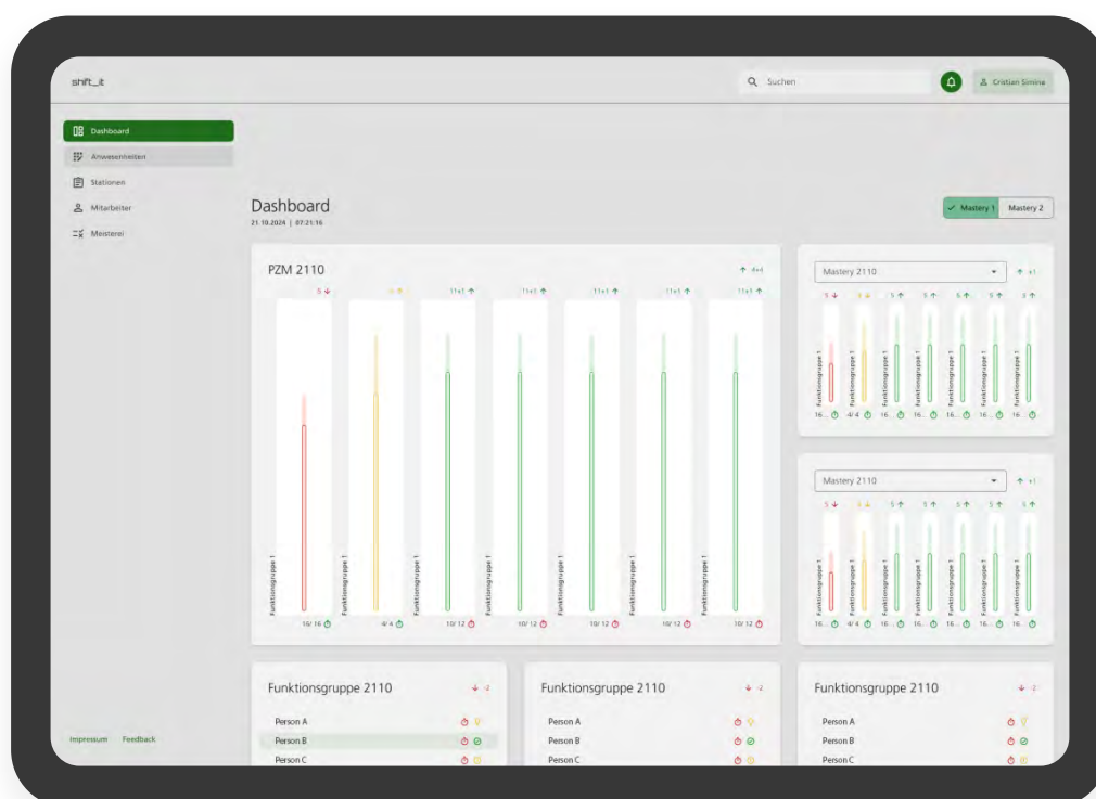
Abbildung 3: Desktop Dashboard
