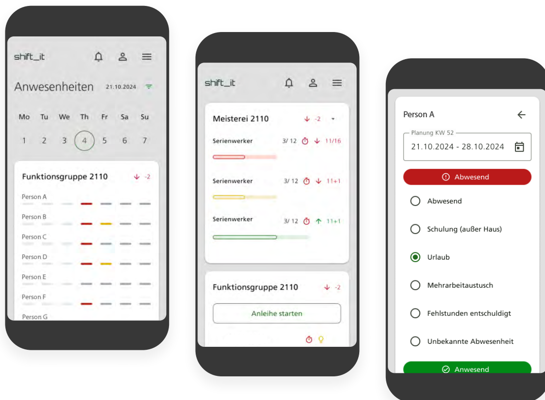
Abbildung 4: Mobile Ansicht
